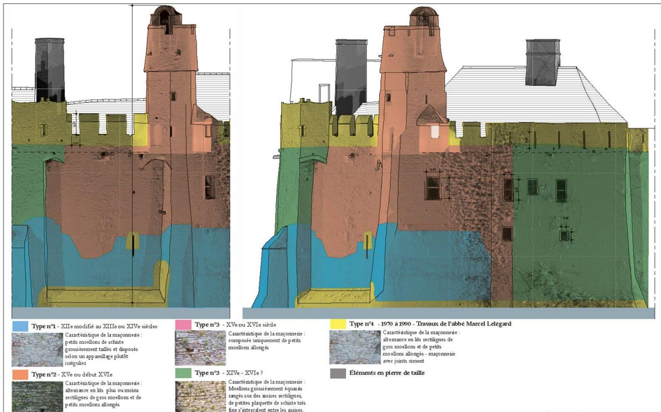
Repérage des typologies de maçonneries du château fort de Pîrou (XII e s.), diagnostic, Arnaud Paquin architecte DPLG, novembre 2018.
